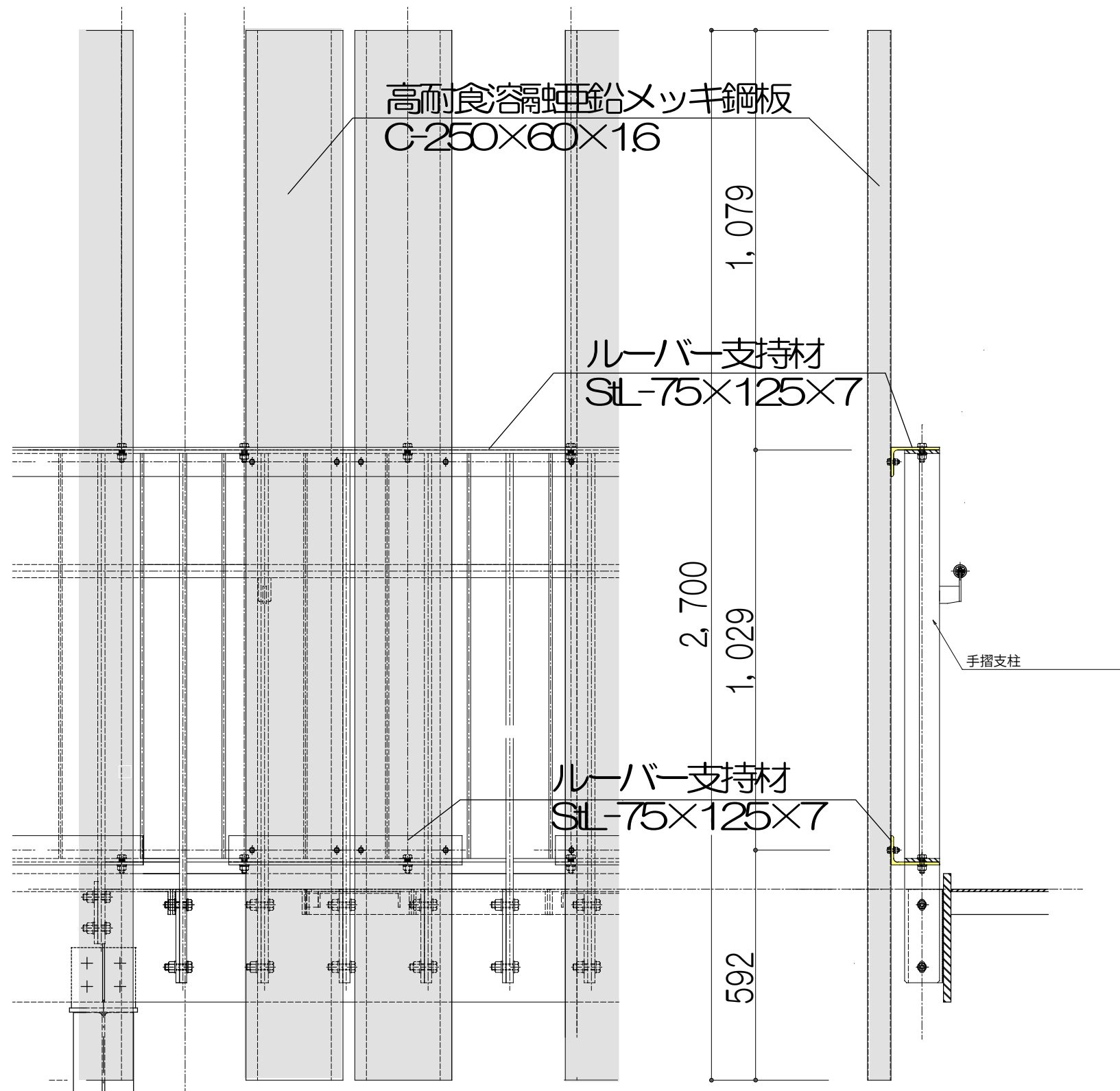
立面詳細図
